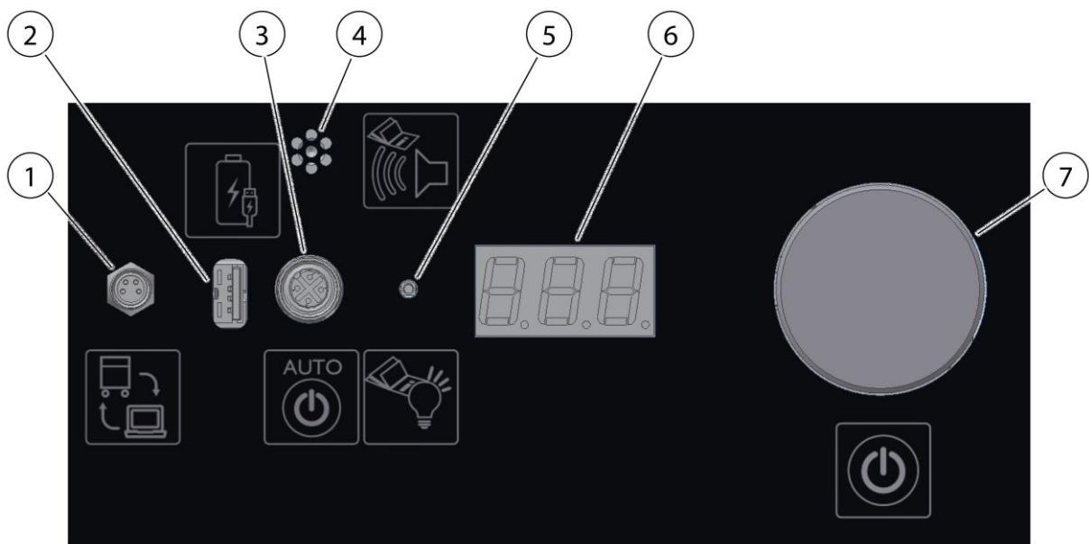
Afb. 8: Bedieningselementen
