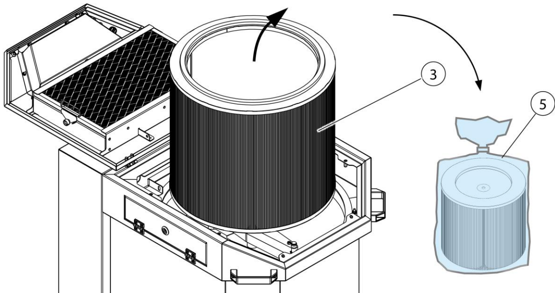
Afb. 12: Filtervervangning – filterpatroon afvoeren
