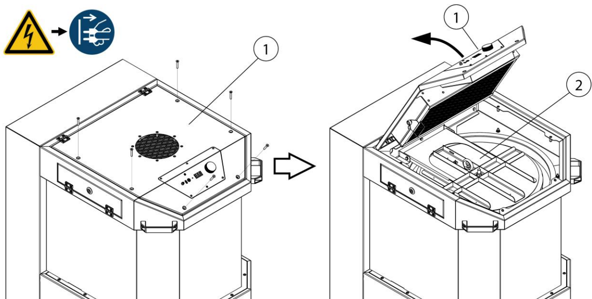
Afb. 10: Filter vervangen – toegang tot de filterpatroon
