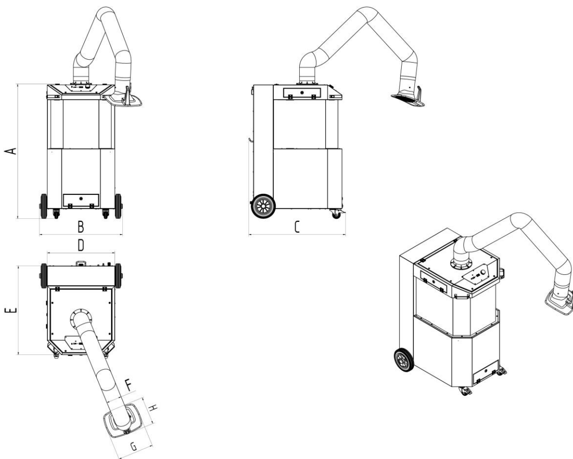
Afb. 14: Maatblad
