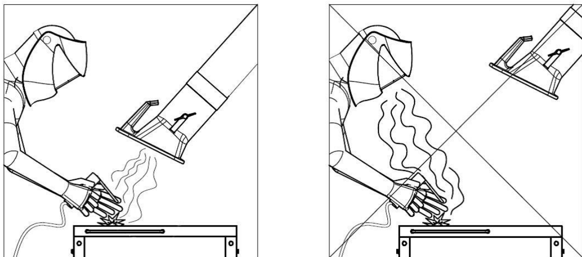
Afb. 9: Positionering van de afzuigkap
